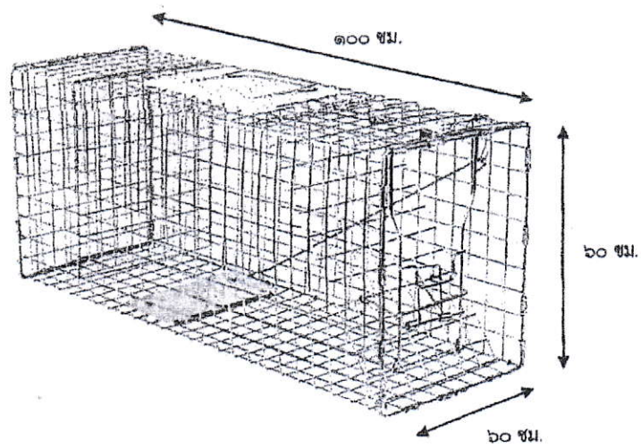
กรงดักจับสุนัข
